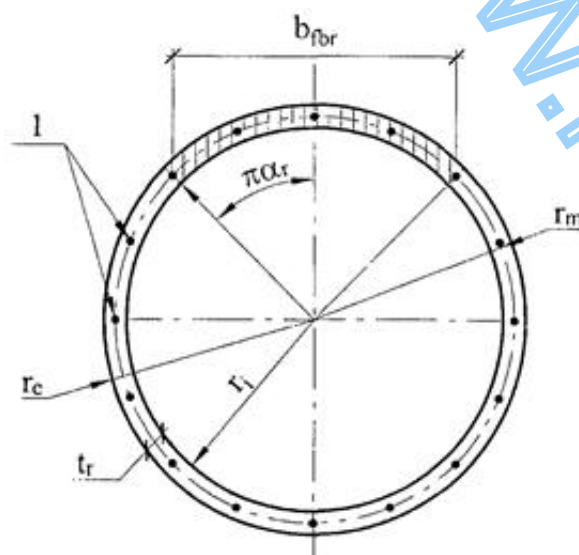
1 - стержневая арматура
