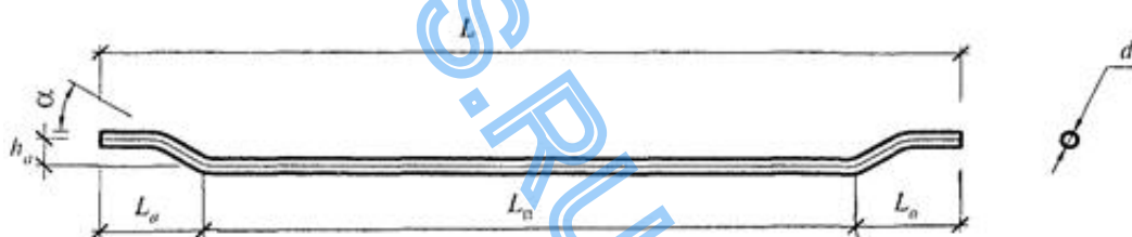
Рисунок Г.3.6 - Форма фибры типа «ФЛА»
